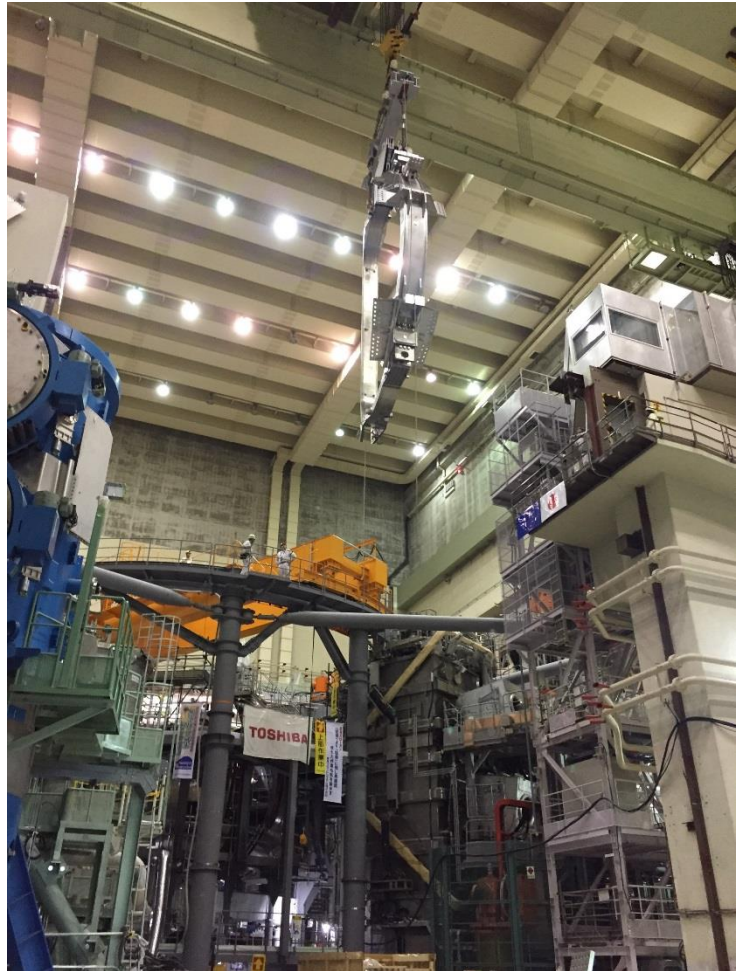
La première bobine et sa structure de liaison sont livrées au Japon et préparées pour une installation sur JT60-SA en juillet 2016. Crédits : A gauche ©
