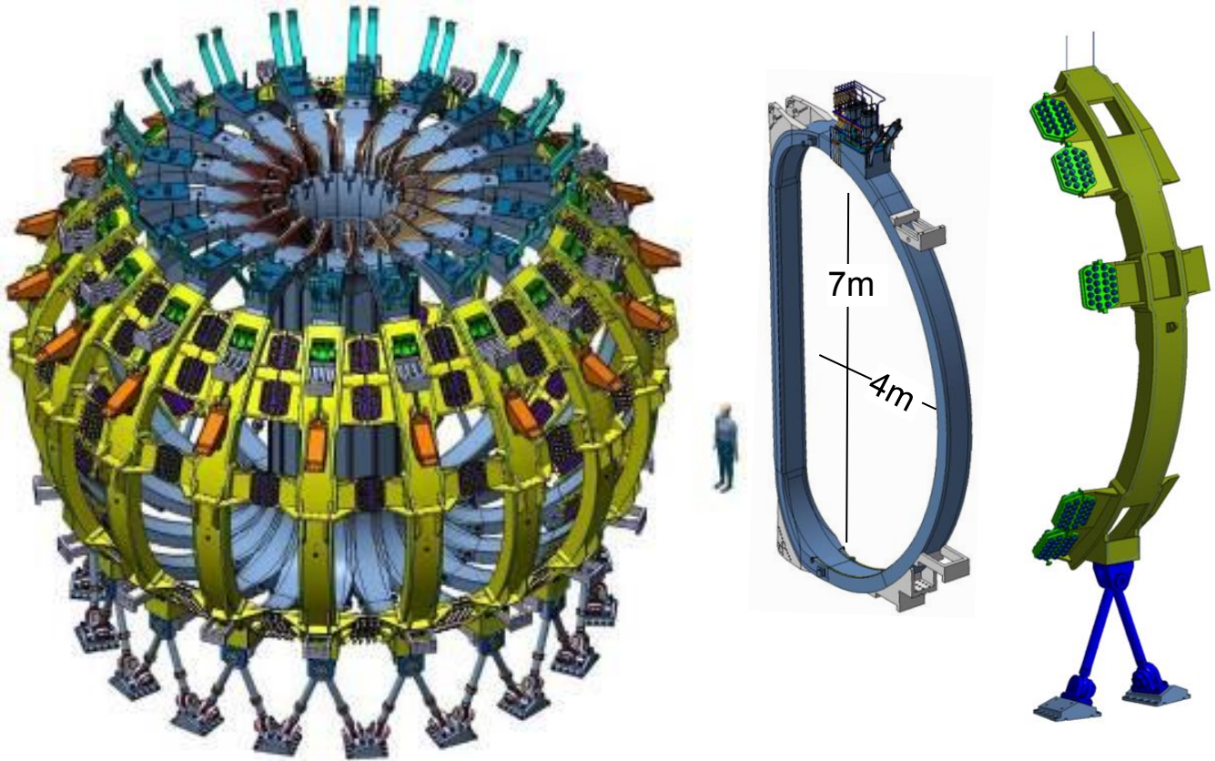
Echelle des éléments du système magnétique de JT-60SA fabriqués en France.
